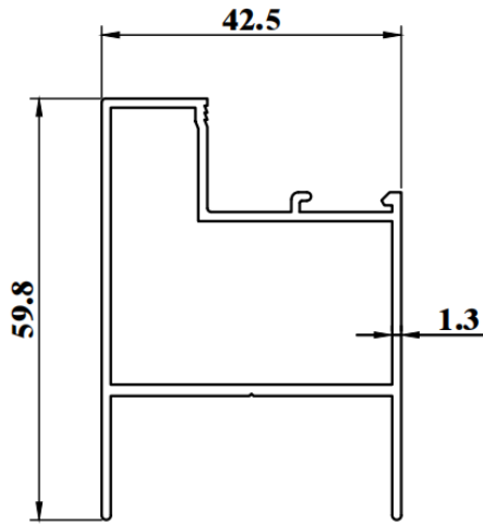
SWD339 WEIGHT : 0.768 KG/M AP : 255.29mm
