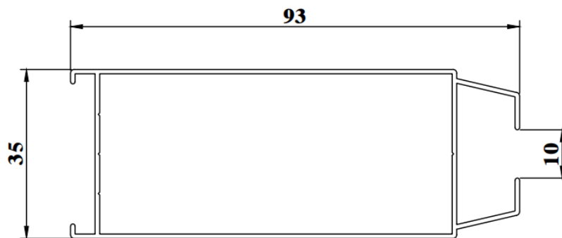
SWD353 WEIGHT : 0.671 KG/M AP : 325.49mm
