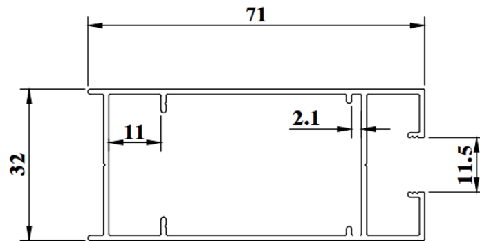
SWD352E WEIGHT : 0.705 KG/M AP : 282.87mm
